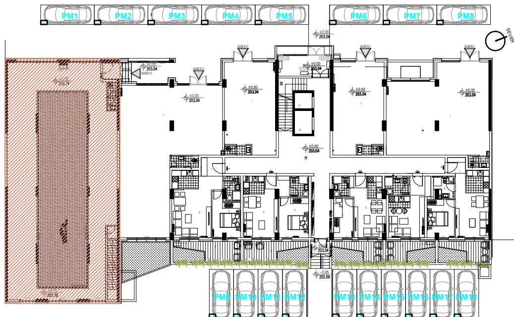
OSNOVA PRIZEMLJA
