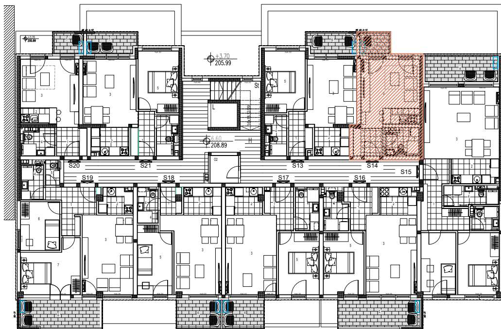
OSNOVA II.SPRATA
