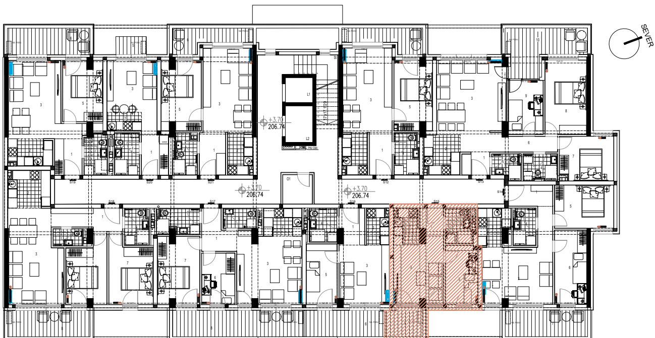
OSNOVA I. SPRATA
