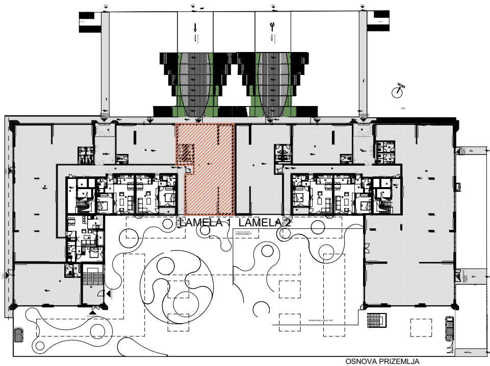
OSNOVA PRIZEMLJA
