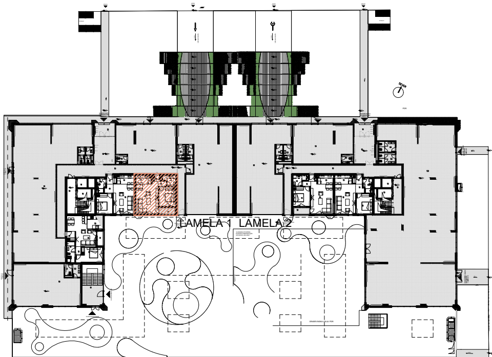
OSNOVA PRIZEMLJA
