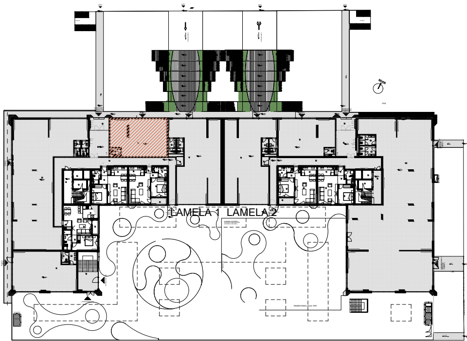
OSNOVA PRIZEMLJA
