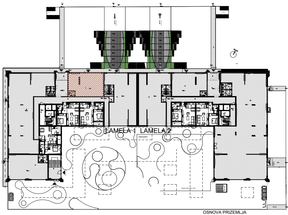
OSNOVA PRIZEMLJA
