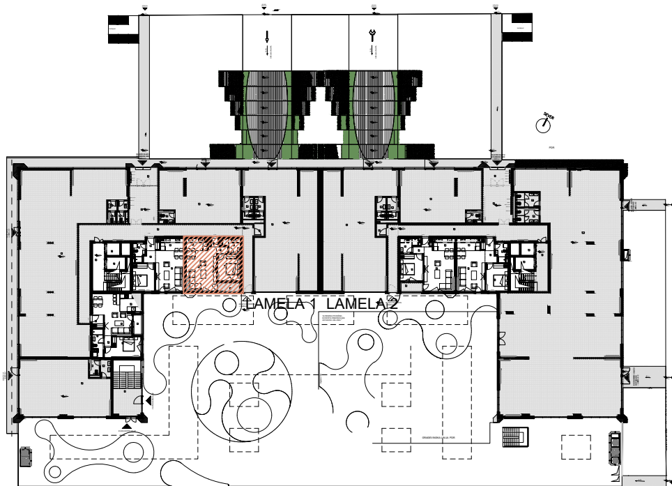
OSNOVA PRIZEMLJA
